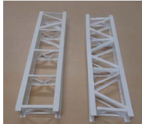
写真 2.4.1 プレートガーダーの模型
